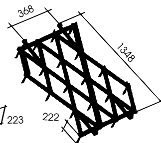
БЗС-1.0.00.000-01 (для жесткой сцепки) М = 33,6 кг
