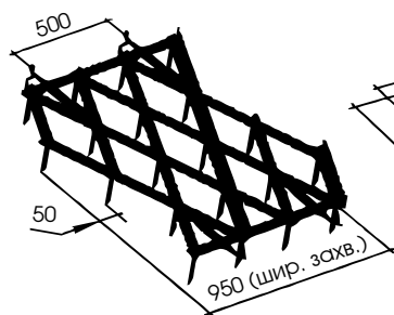
БЗС-1.00.000 М = 33,8 кг
