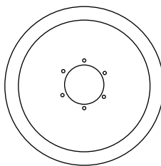
СП6Д.14.192 Диск сошника
