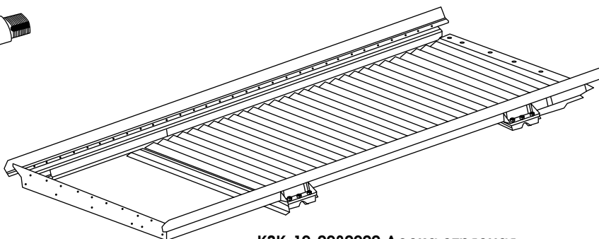
КЗК-12-0280200 Доска стрясная
