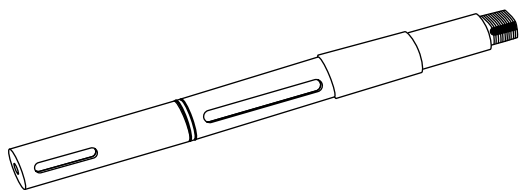
КЗК 0207608 Вал домолачивающего устройства
