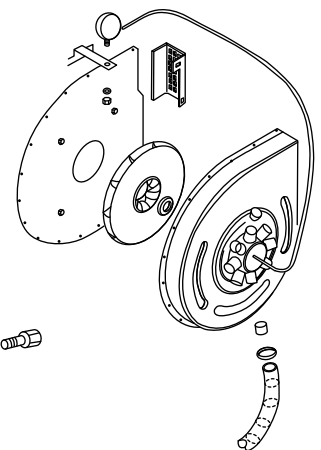
083.601 Семяпровод
