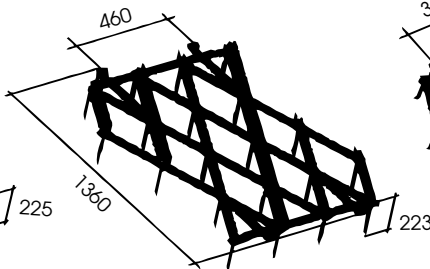
БЗС-1.0.00.000-05 (для жесткой сцепки) М = 46,9 кг
