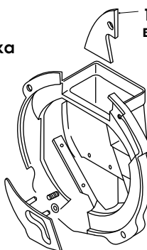
040.219 Прикатывающее колесо
