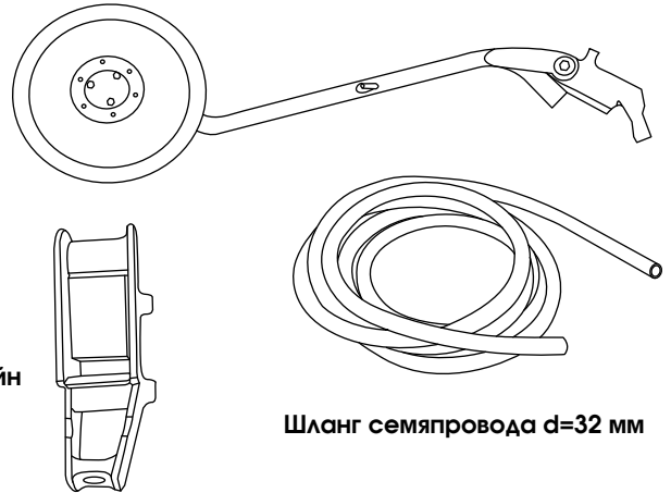
СП6Д.14.200/100сб Сошник дисковый длинный и короткий
