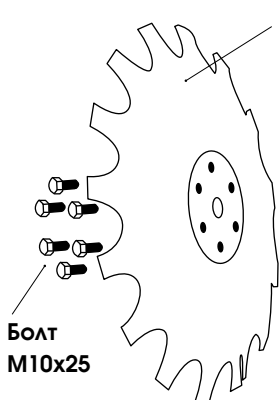
53-4107 Диск 510х4
