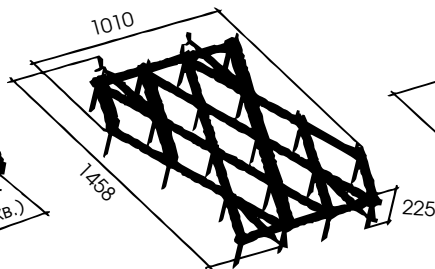
БЗС-1.0.00.000-02 М = 48 кг
