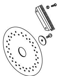
10034124 Чистик высеивающего диска
