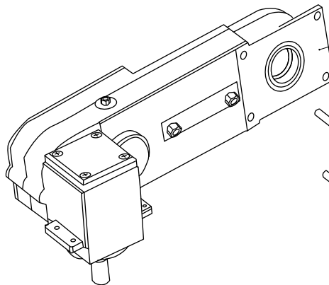
КПС-4-0515200-01 Редуктор привода
