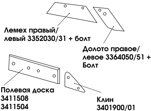
Грудь отвала правая/левая 3451000/01
